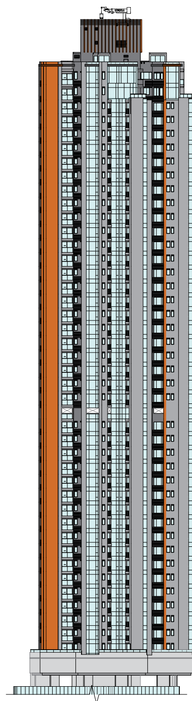
ELEVATION PLAN 3 立面圖 3
