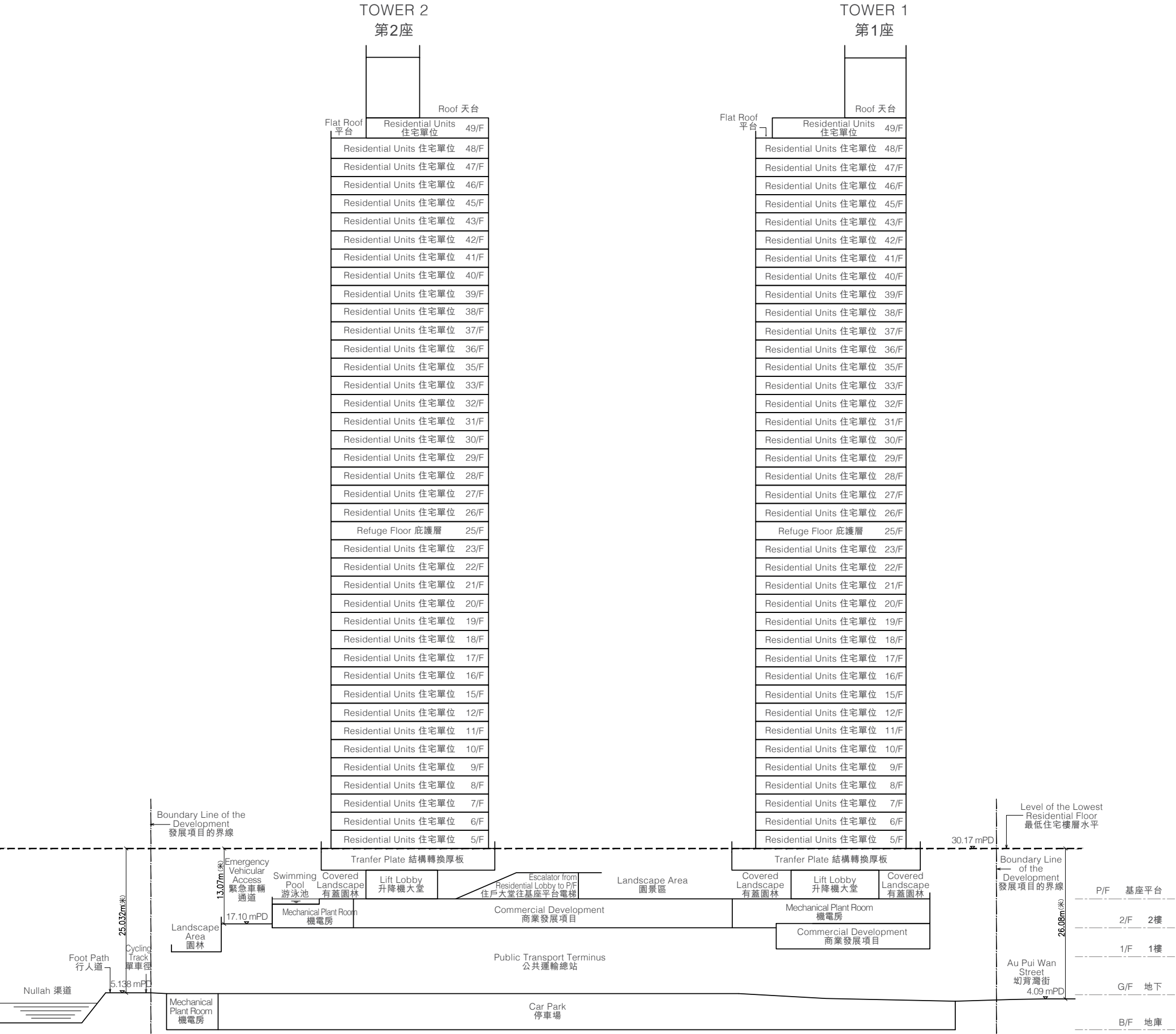
CROSS-SECTION A-A 橫截面圖 A-A
